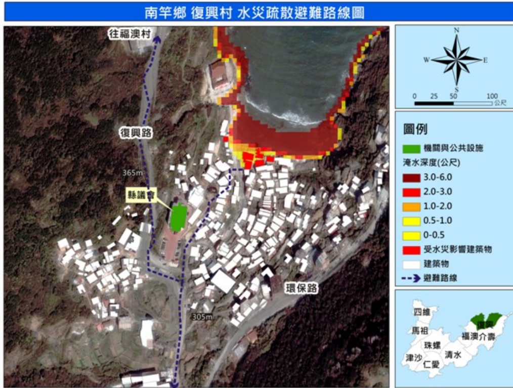
圖2-1 復興村颱風災害避難路線圖
